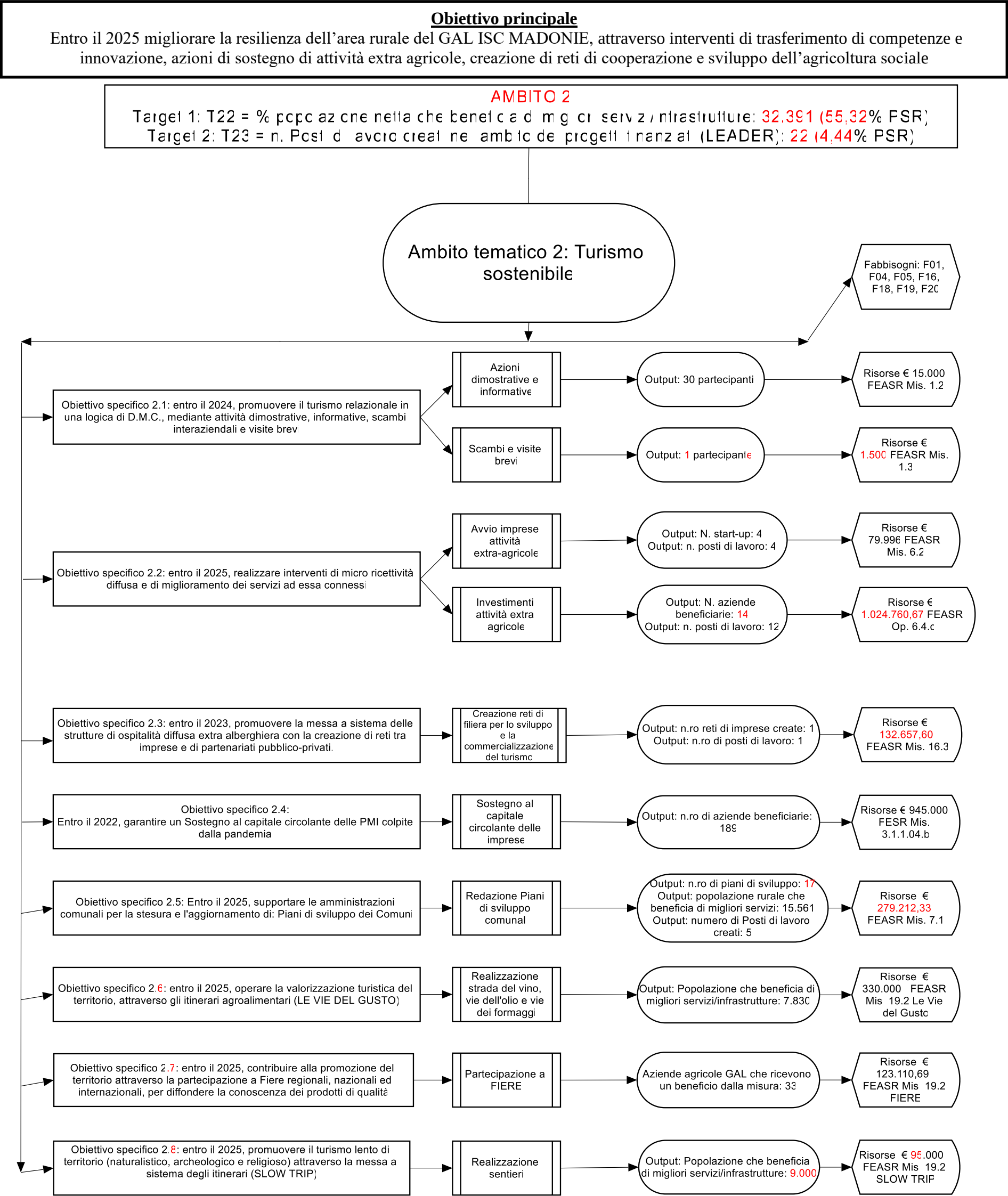
Figura 3 REV. 4.2 – Quadro logico degli interventi nell’ambito tematico “Turismo sostenibile”
